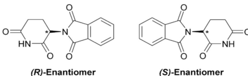
Figura 4: Els dos enantiòmers de la talidomida
